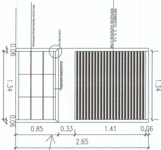
VISTA FRONTAL A PANEL E BALCÃO DE APOIO PARA CHÁ / CAFÉ
